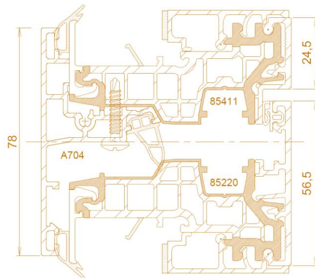
CONFIG. DORMANT / OUVRANT
