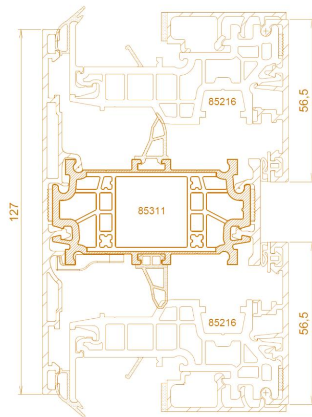
CONFIG. OUVRANT / MENEAU
