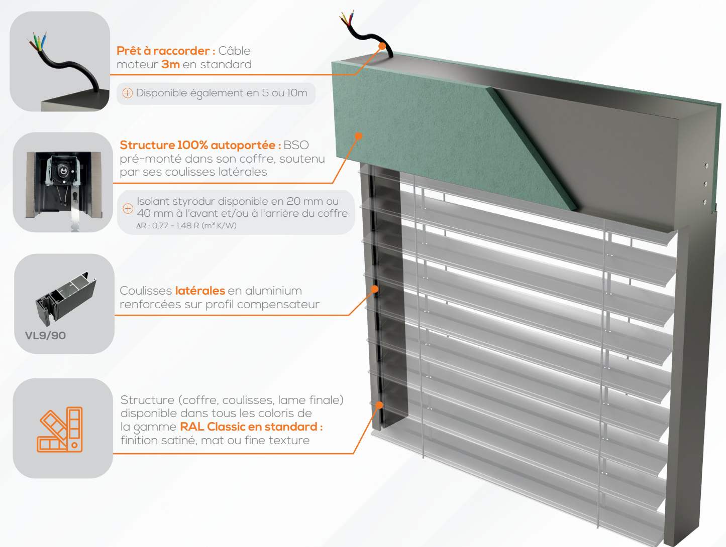
Comfort System CP20 avec isolant avant et arrière
